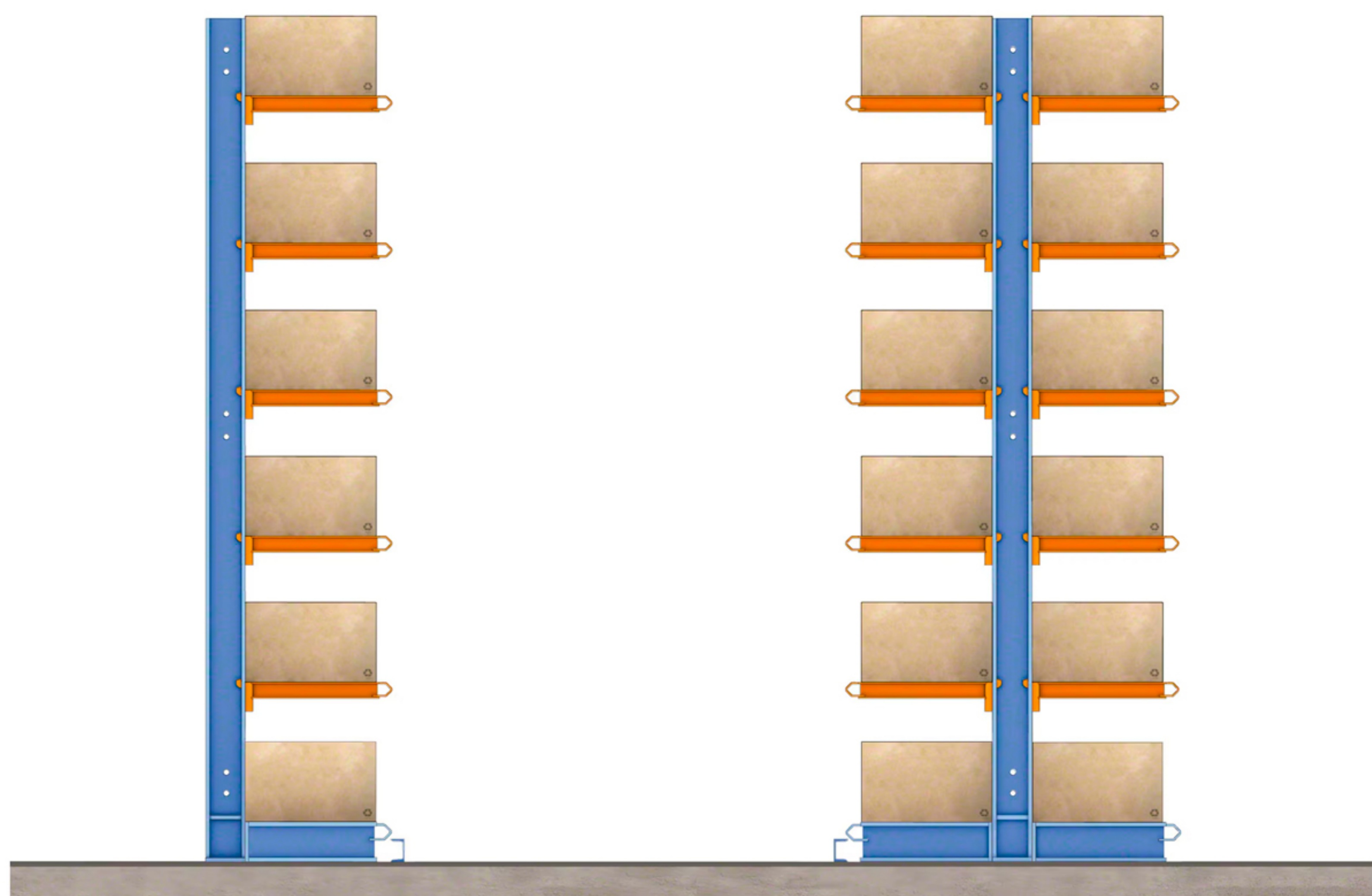
Cantilever Personalizado
